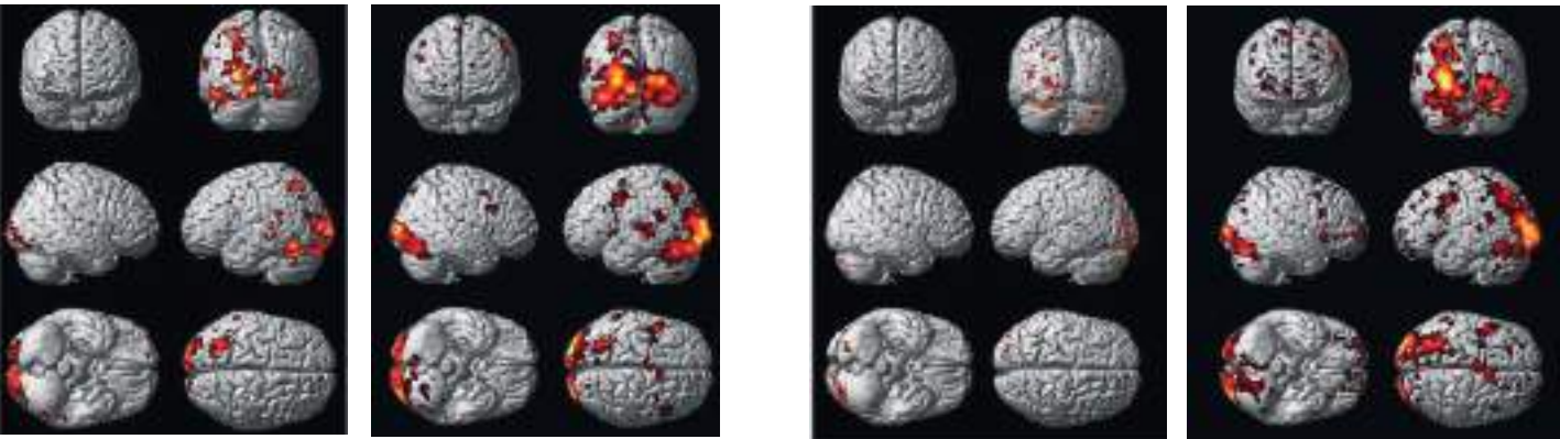
Fig. 1: imagens de renderização tridimensional de correlações entre o desempenho em (a) registro e (b) tarefa de recuperação de memória verbal.
